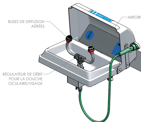
VUE ISOMÉTRIQUE (COUVERCLE OUVERT)
