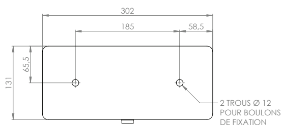
DÉTAILS DE FIXATION MURALE ÉCHELLE 1:5
